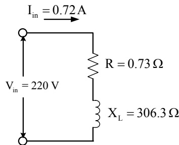
รูปที่ 8 วงจรสมมูลทางด้านอินพุตของหม้อแปลงอโต้ขณะยังไม่จ่ายโหลด
