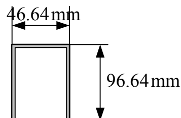
รูปที่ 7 ภาพตัดแกนเหล็กรวมจำนวนของหม้อแปลงออโต้ที่เผื่อจำนวนข้างละ 2 mm รวมรัศมีลวด ตัวนำ 1.32 mm โดยด้านบนและล่างเผื่อจำนวนด้านละ 5 mm ด้วย
