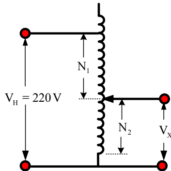
รูปที่ 6 แสดงพารามิเตอร์ต่างๆ ของหม้อแปลงแบบออโต้ที่ใช้คำนวณ
