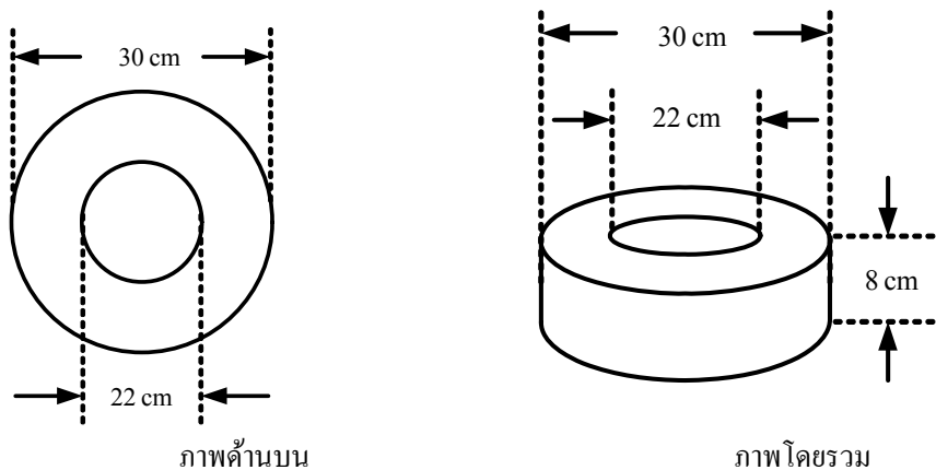
รูปที่ 1 ขนาดแกนเหล็กชนิด Electrical iron ที่ใช้พันขดลวด
